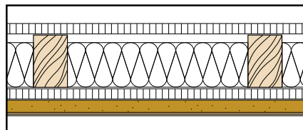
Holzständerwand
