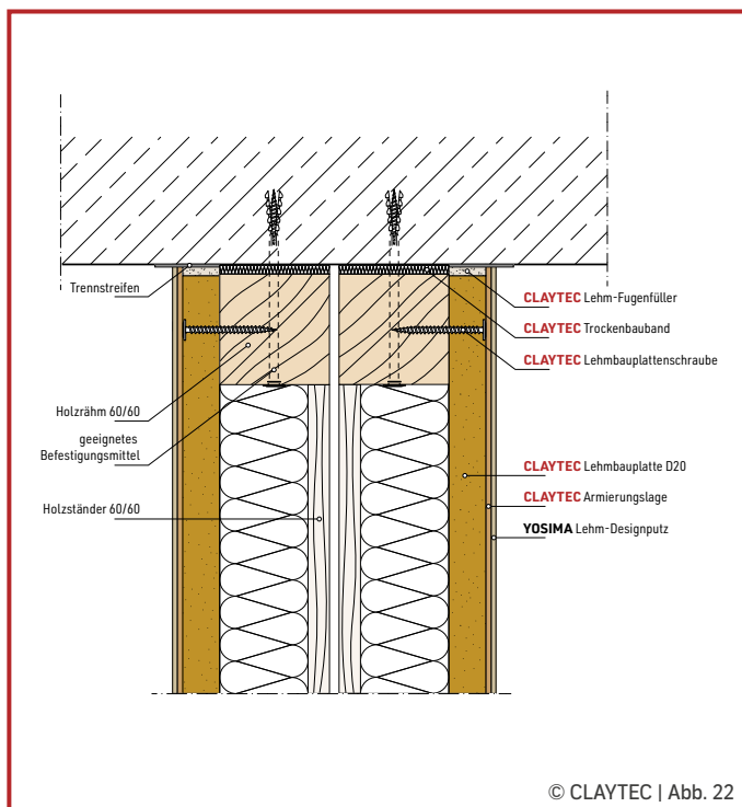
Holzkonstruktion Doppelständer Anschluss an Massivdecke
