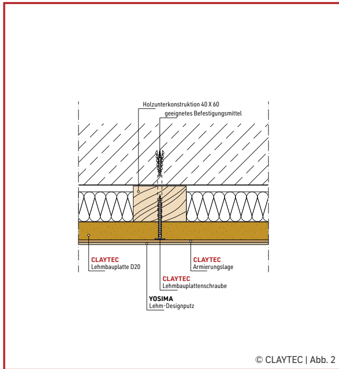
Holzkonstruktion Vorsatzschale direkt befestigt
