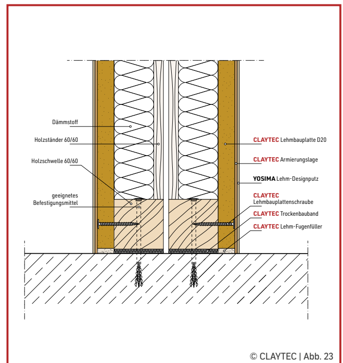
Holzkonstruktion Doppelständer Anschluss an Massivboden
