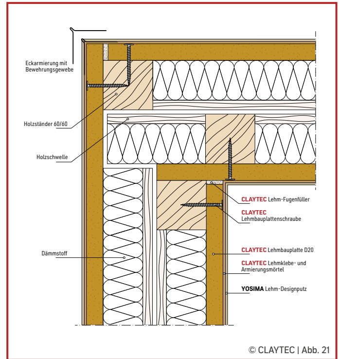
Holzkonstruktion Doppelständer Eckanschluss
