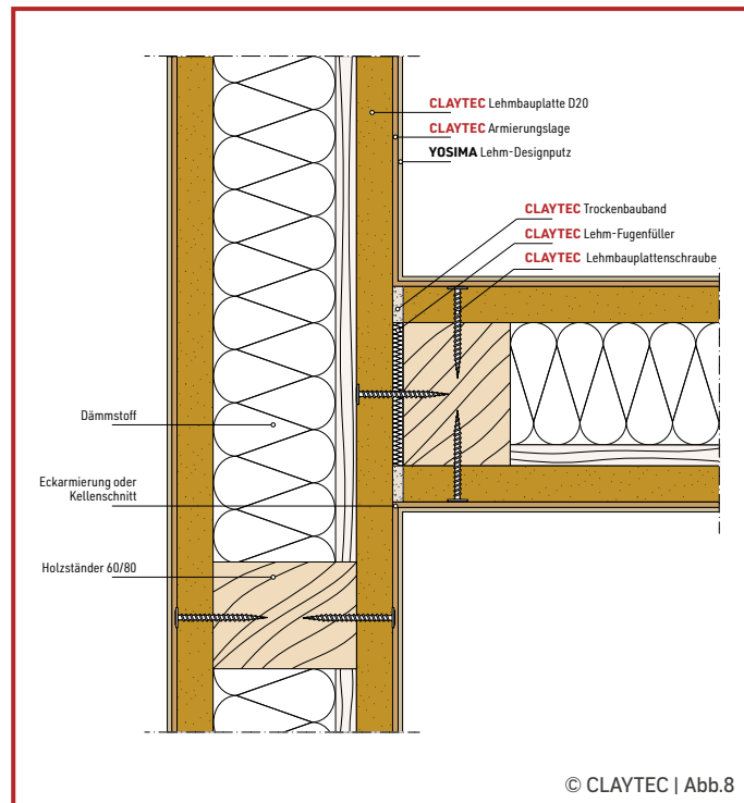
Holzkonstruktion Anschluss an Trockenbauwand
