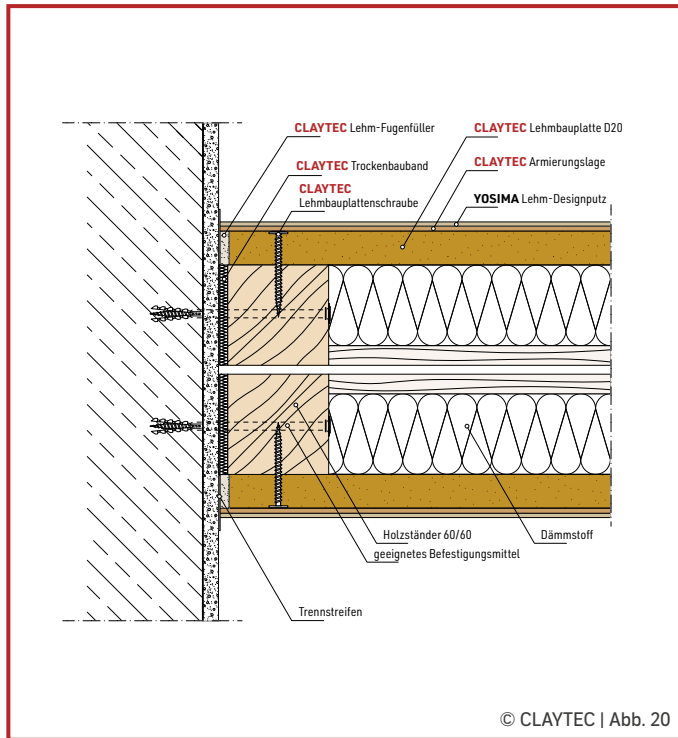
Holzkonstruktion Doppelständer Anschluss an Massivwand
