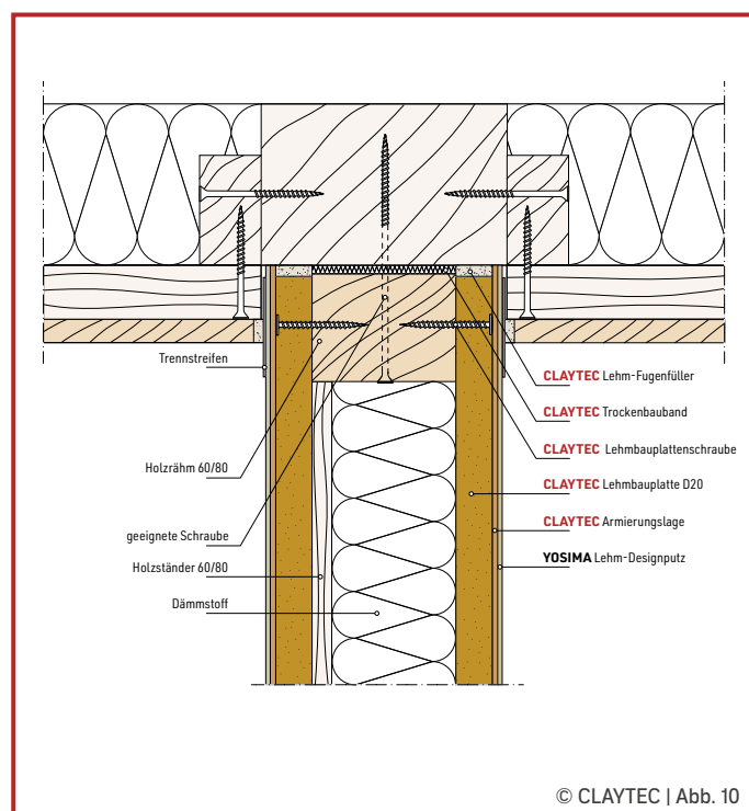
Holzkonstruktion Anschluss an Holzbalkendecke
