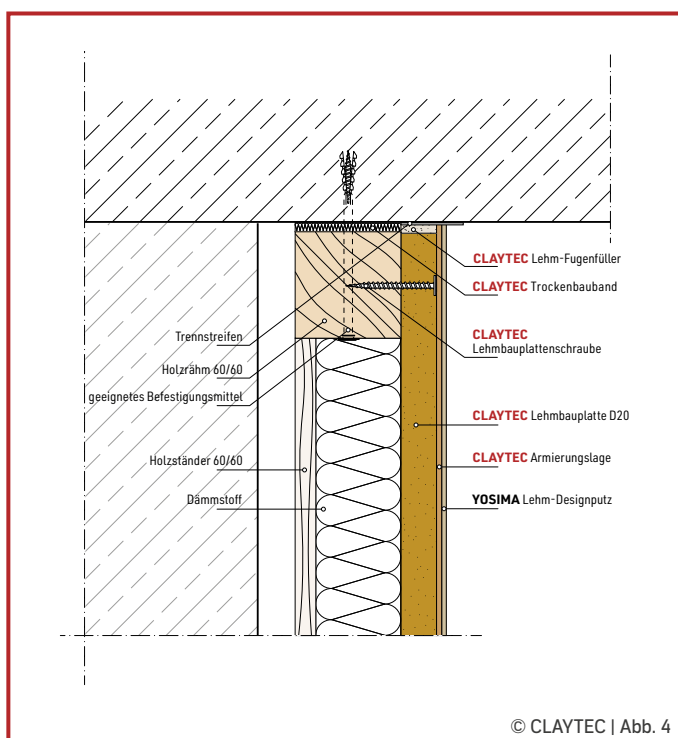
Holzkonstruktion Vorsatzschale Anschluss an Massivdecke
