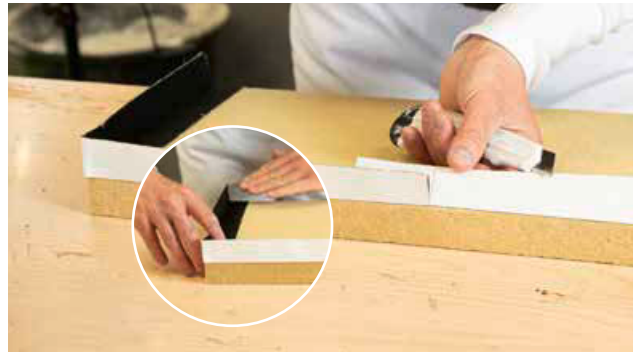
3 Die STEICOmulti tape black Klebestreifen mind. 5,0 cm überlappen, so dass sich eine dichte, dreiseitige Wanne ausbildet
